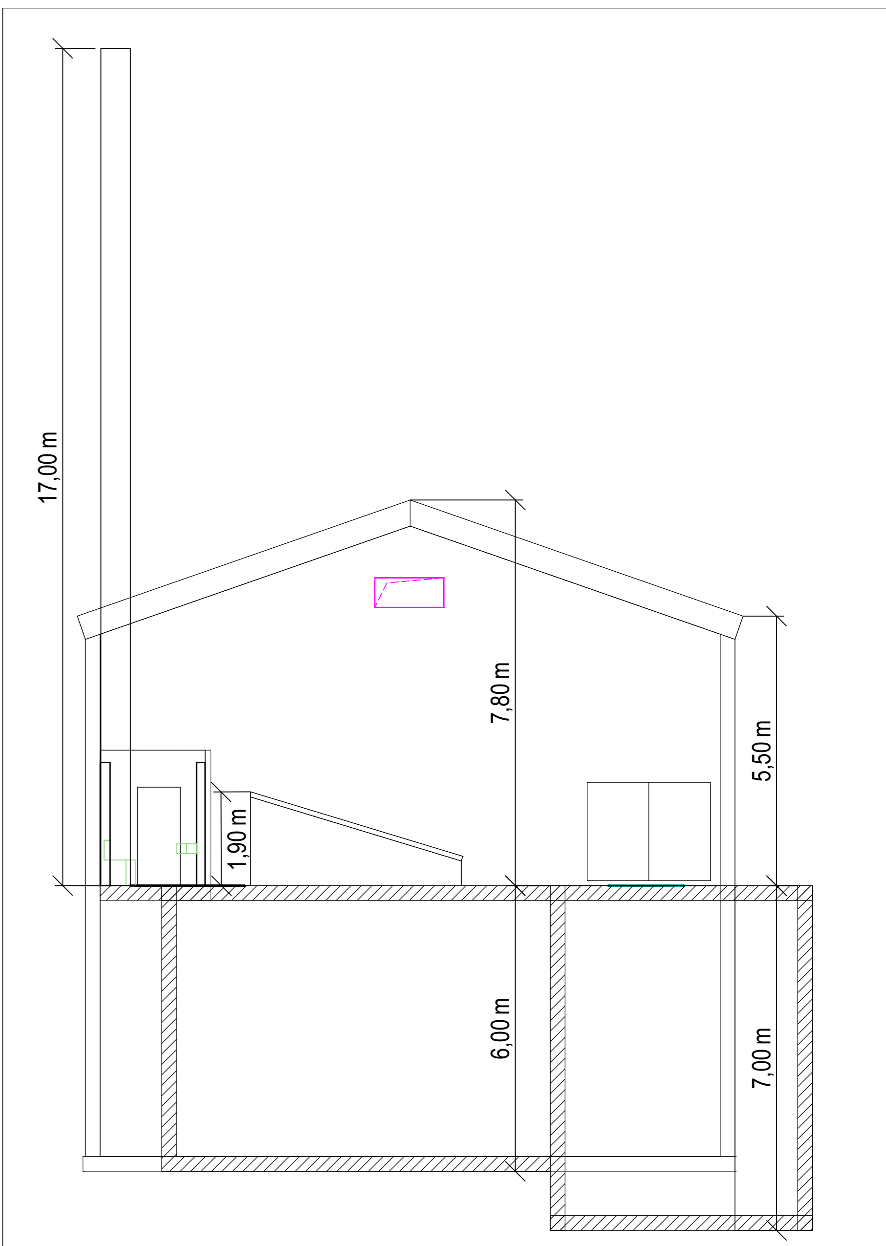
Schnitt 1:75
